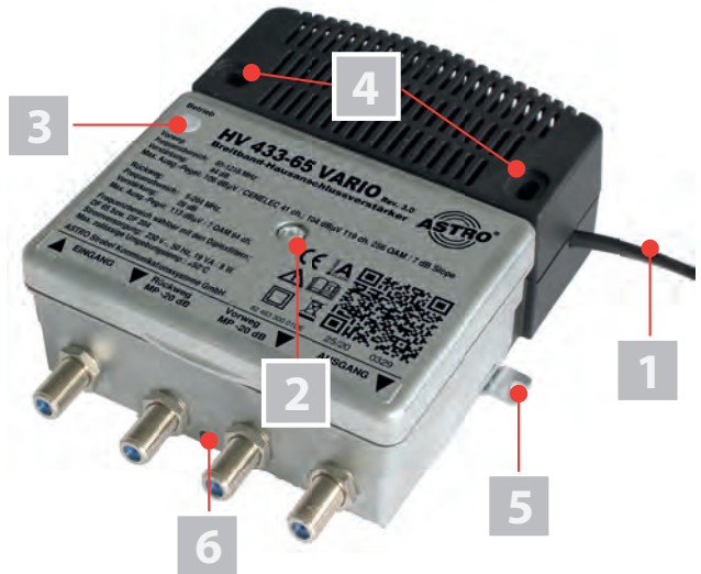
Bild 1: Verstärker HV 433-65 Vario (HV 433-85 Vario ähnlich)
